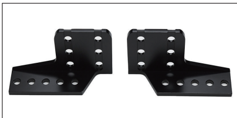
バランスステー MW 寸法：長さ 84.5mm、高さ 50mm、重さ約 39g
