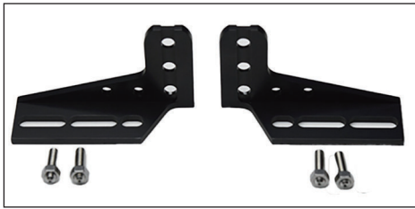
バランスステー M 寸法：長さ 84.5mm、高さ 50mm、重さ約 30g
